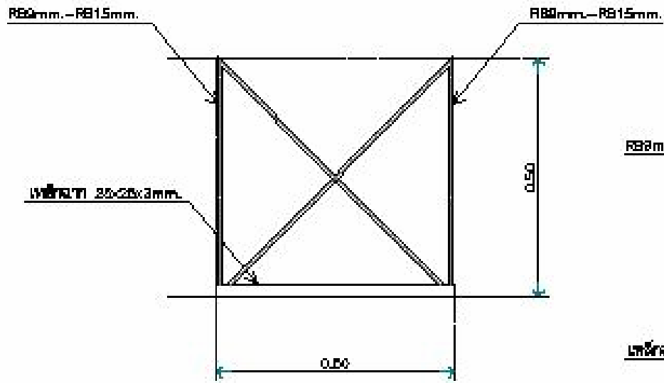
รูปด้านข้าง ขนาดจริง 1:10
