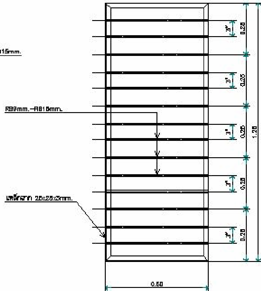
รูปด้านบน ขนาดจริง 1:10
